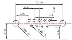
PCB布局 (PCB Layout)
